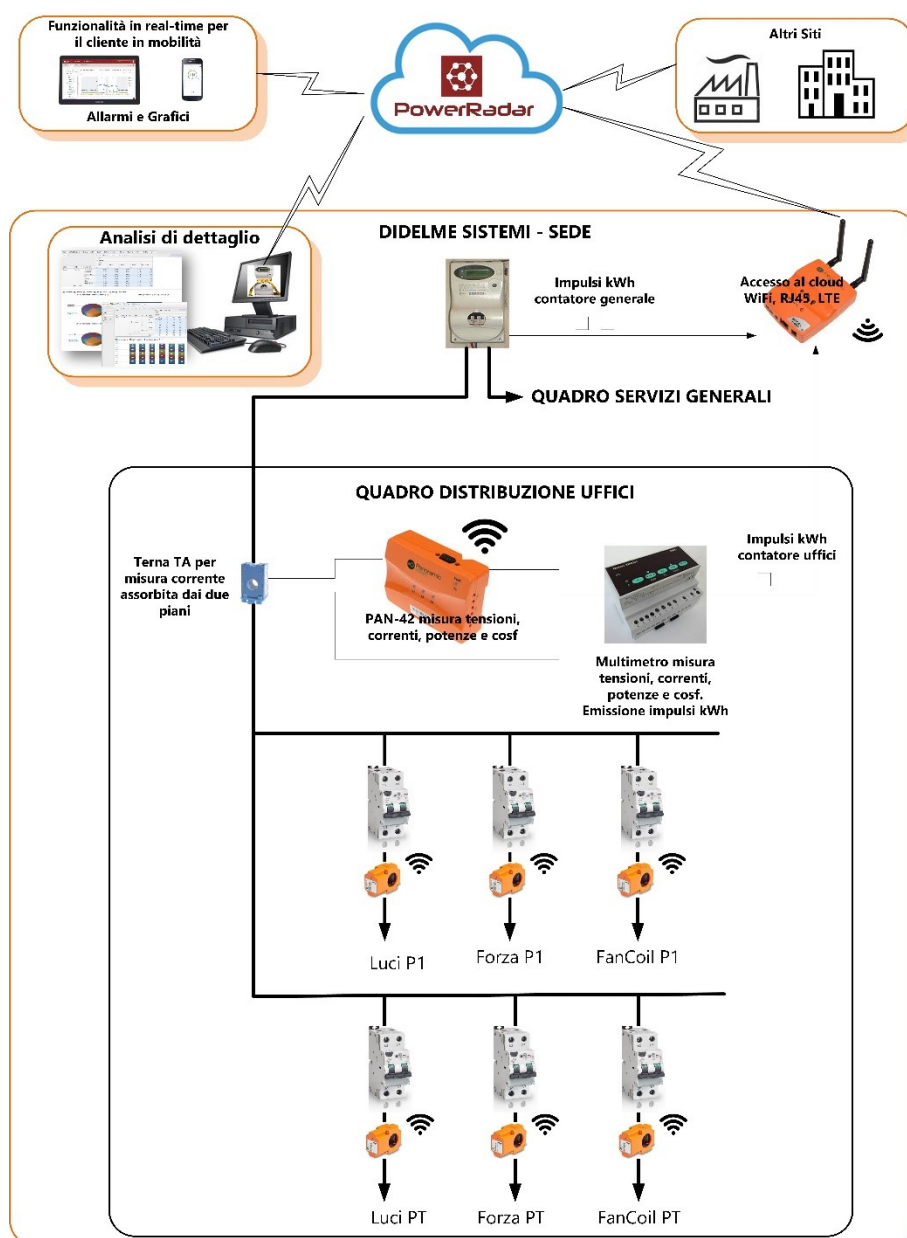
Figura 1 – organizzazione dei sensori e dei segnali impulsivi
